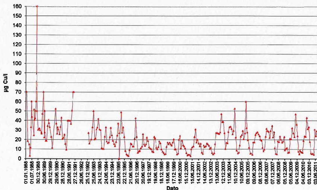
Figur 3. Kobberkonsentrasjoner ved utløpet av Langvann ved Hellarmo 1988-2011.
